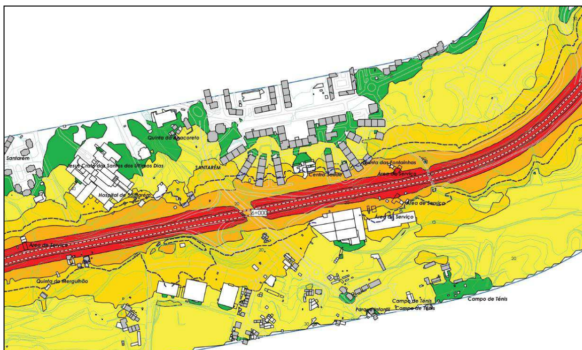
Figura 4-4 – Extrato do MER do IC10/EN3 para o indicador L_n
