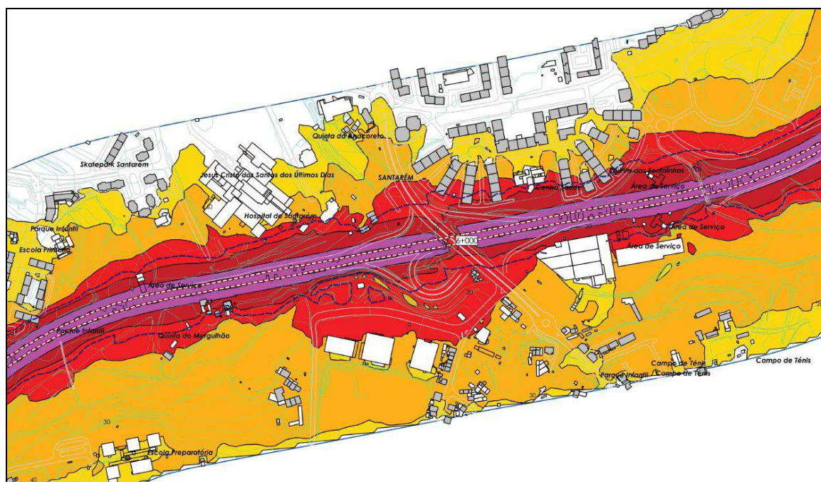
Figura 4-3 – Extrato do MER do IC10/EN3 para o indicador L_{den}
