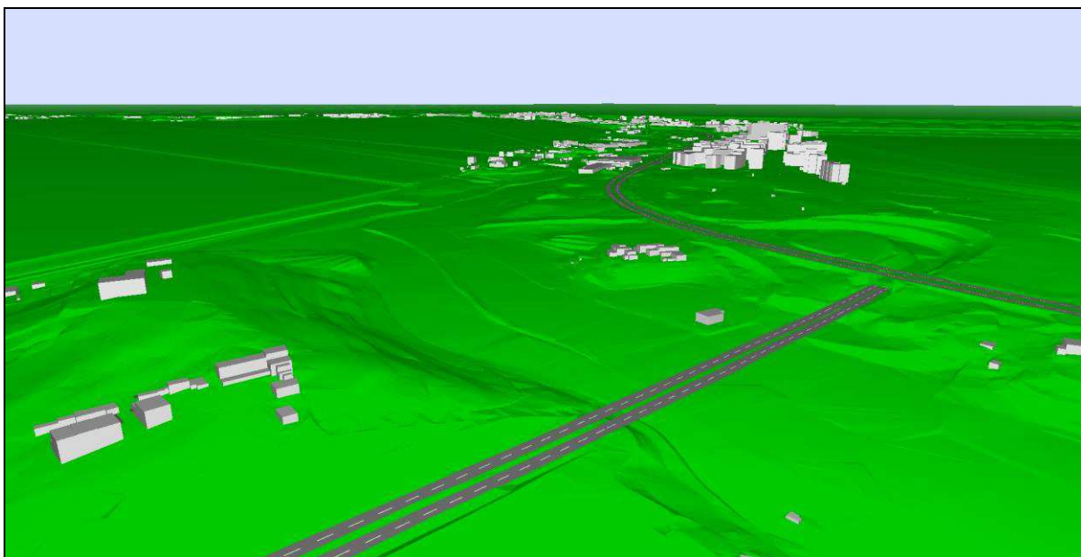
Figura 4-1 – Modelo digital do terreno construído com base nos elementos cartográficos, já com os troços do IC10/EN3 e do IC10 implantados
